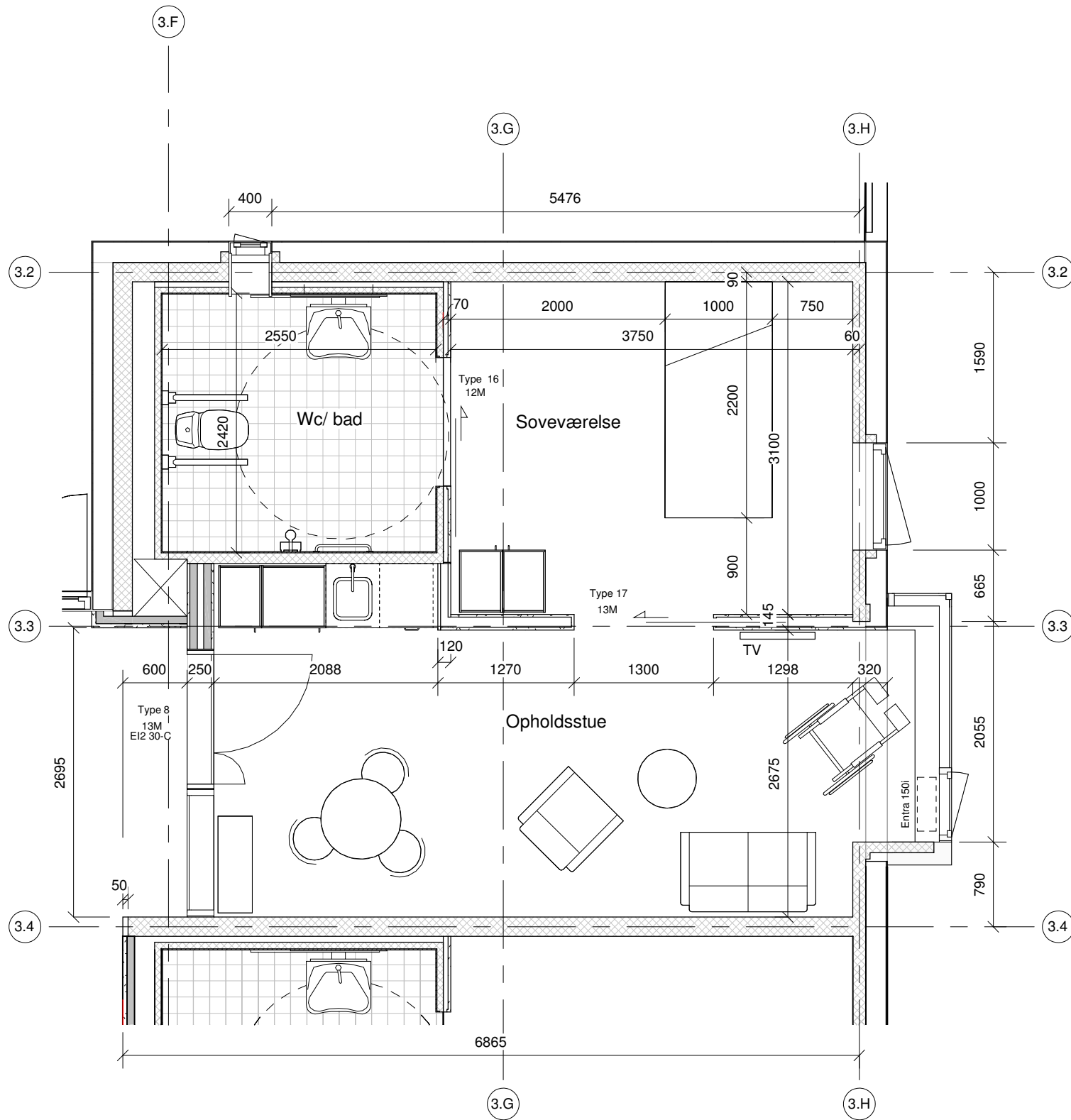
Bolig type 2 - m. vindue
