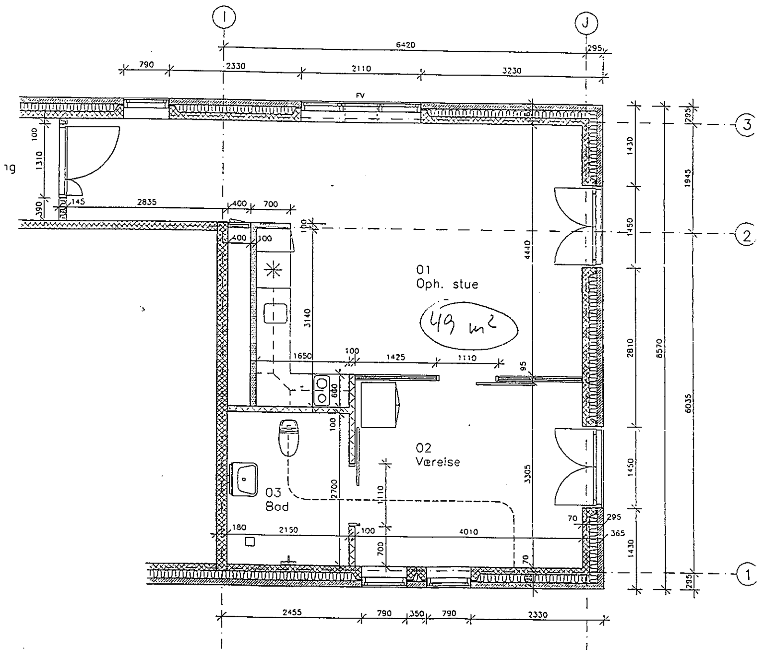
Plan, boligtype B 1.9-2.9
