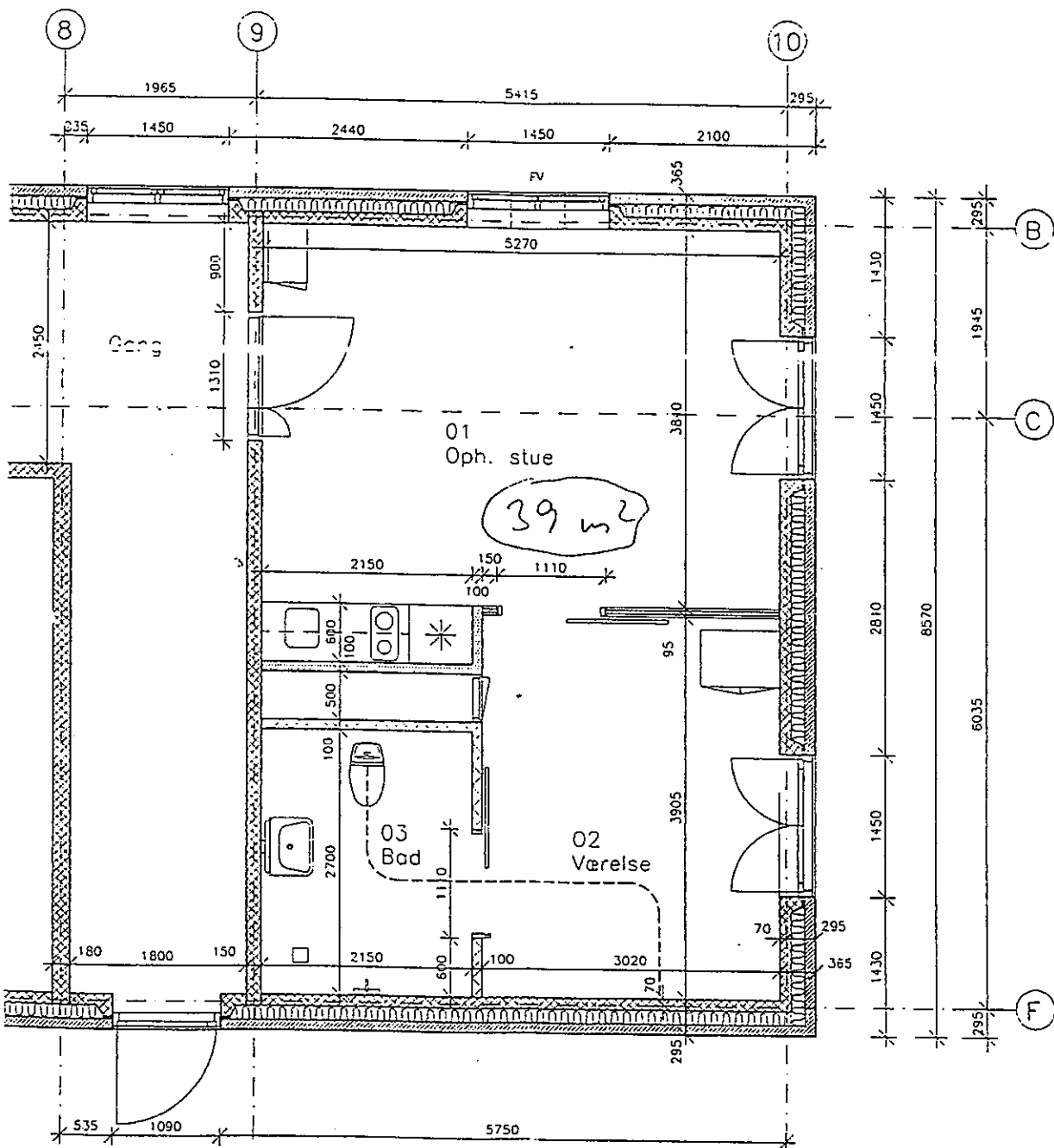
Plan, boligtype B 0.1-1.1-2.1
